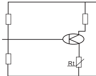
(A) 接在发射极电路
